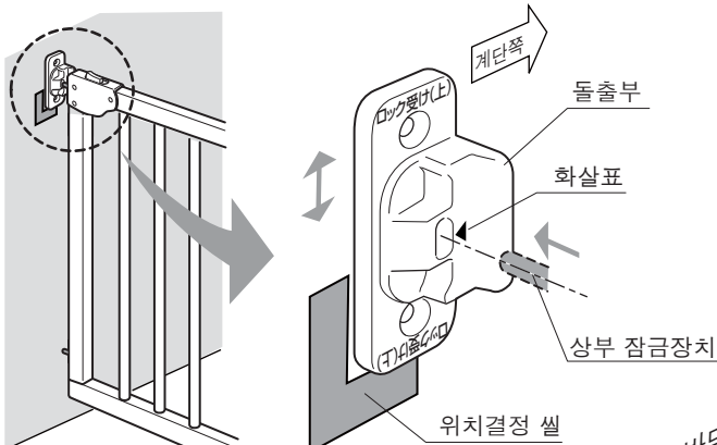
잠금고정 (상)
