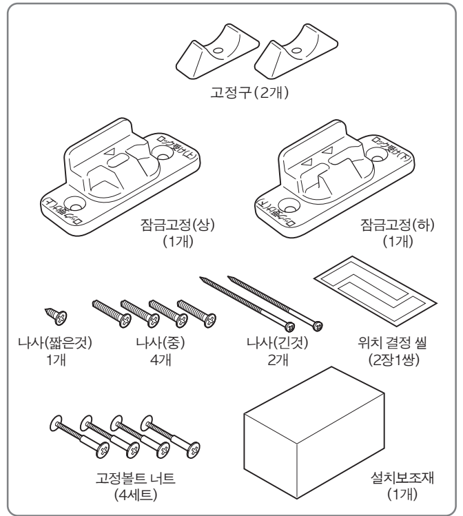
부속부품
