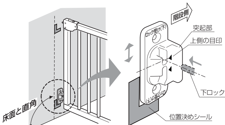
ロック受け(下)
