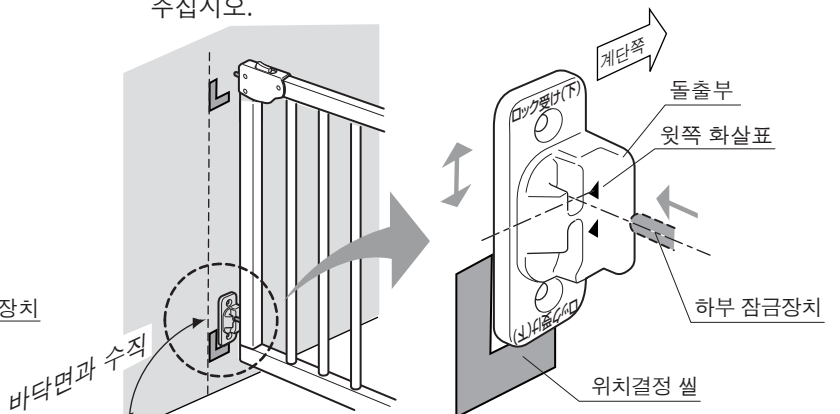
잠금고정 (하)
